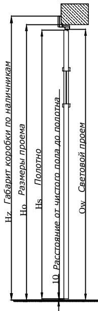
Размеры дверей маятниковых металлическая угловая и обжимная коробка для двустворчатой двери: наличник 80мм
